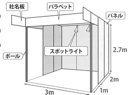
【標準小間仕様図】※1小間の場合。
